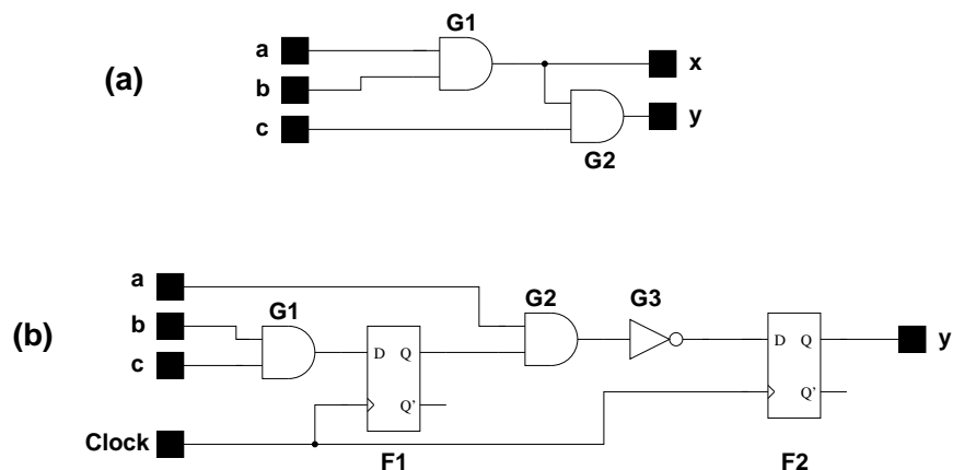
Abbildung 8: Verzögerung in Schaltungen
