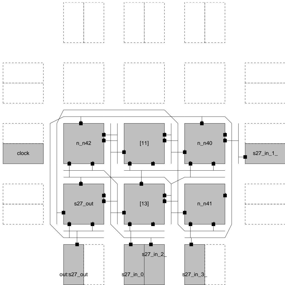
Abbildung 11: Platzierte und verdrahtete Beispielschaltung
