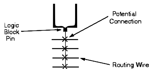
Abbildung 5: Aufbau eines Verdrahtungskanals
