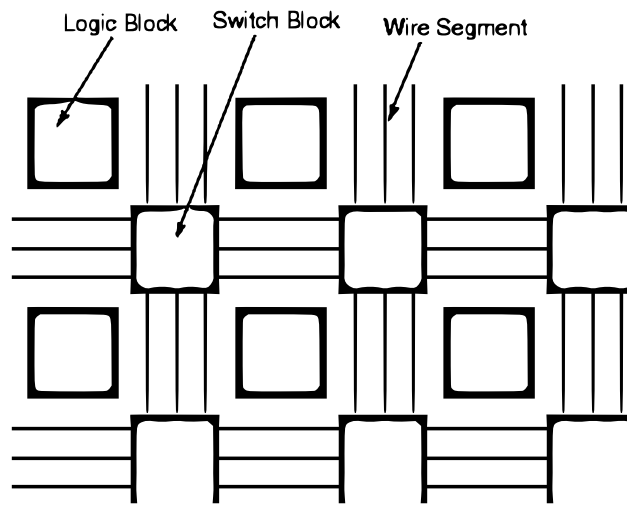
Abbildung 6: Leitungslängen in Kanälen
