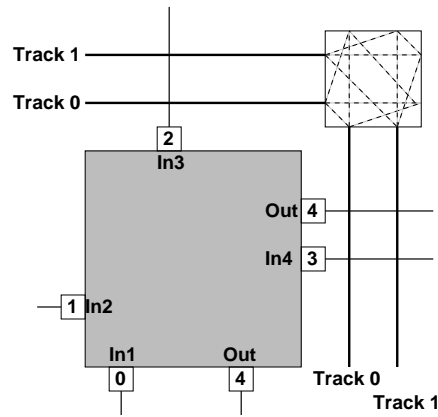
Abbildung 12: Block und dazugehörige Verdrahtungskanäle
