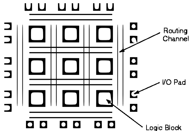
Abbildung 1: Struktur des FPGAs
