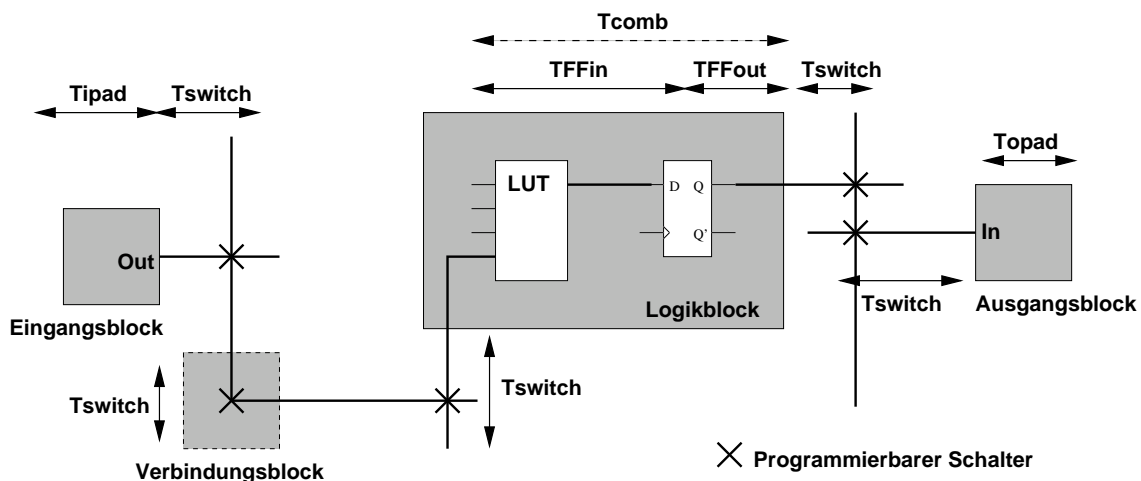
Abbildung 9: Signalverzögerungen
